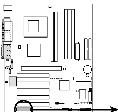
A7A266-E Audio Modem Riser (AMR) Slot
